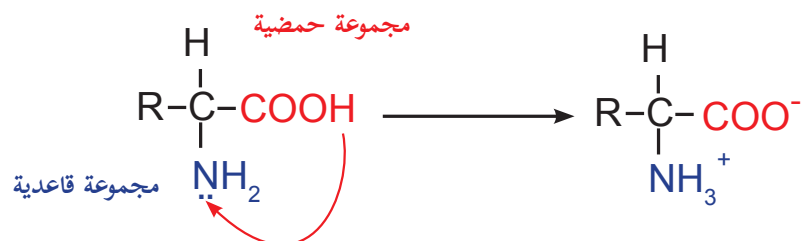
الشكل (8-3): تَشكُّل الأيون المزدوج في الحمض الأميني
