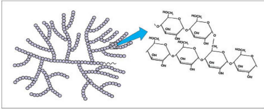
الشكل (3-6): مقطع من سلاسل الغلايكوجين (ليس للحفظ)
