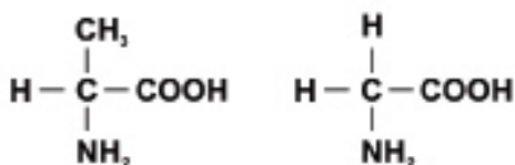
alanine ألانين
